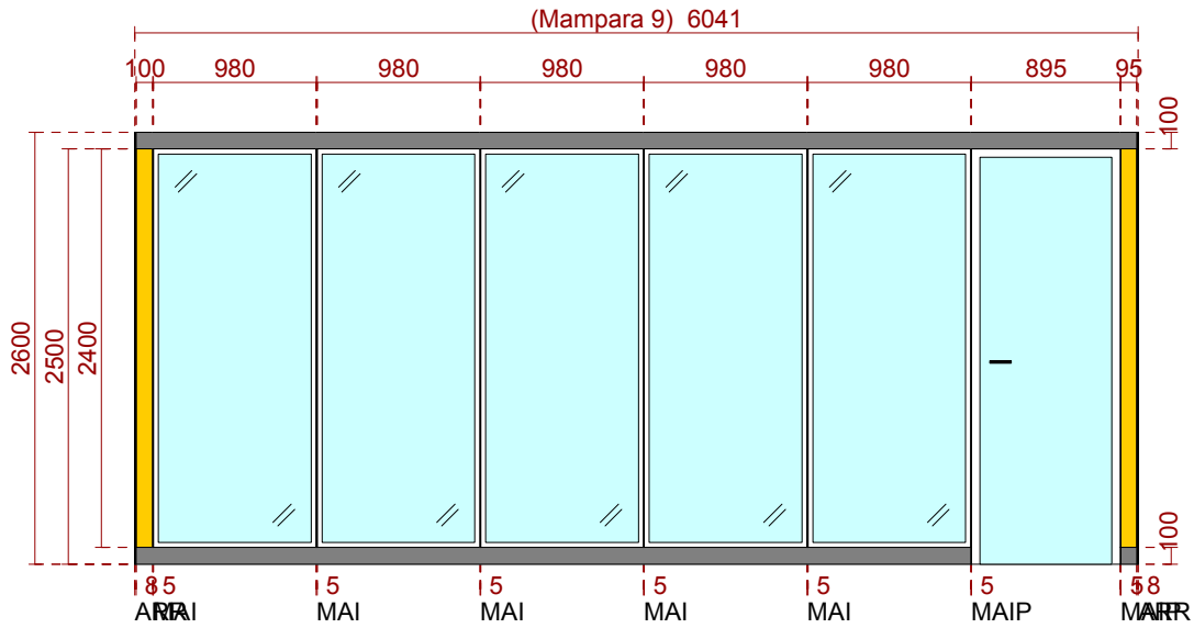
MAMPARA TOTALMENTE ACRISTALADA CON PUERTA DE VIDRIO
