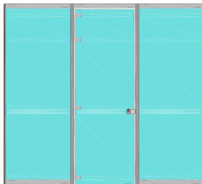
MODELO 1 PUERTA DE VIDRIO SUELO- TECHO CON BATIENTE CORTADO A INGLETE
